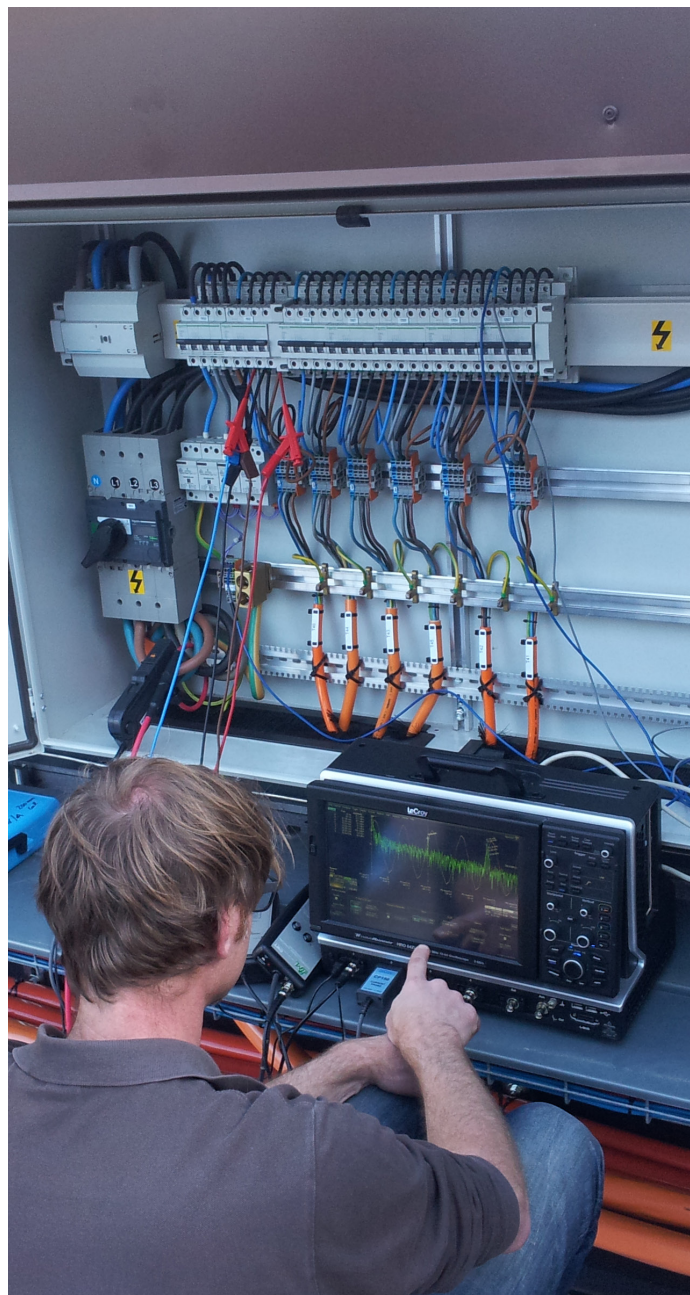
Dominique Roggo, professeur à la HES-SO Valais-Wallis, pendant la mesure de perturbations sur une installation photovoltaïque. Photo: D. Roggo
