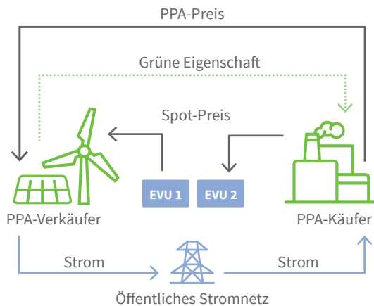
Abbildung 28: Finanzielles PPA
