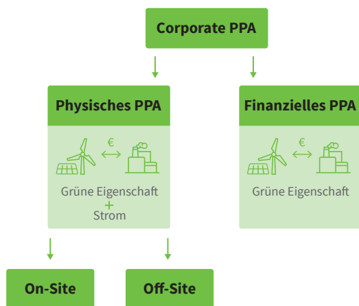
Abbildung 19: Grundsätzliche Corporate-PPA-Formen
